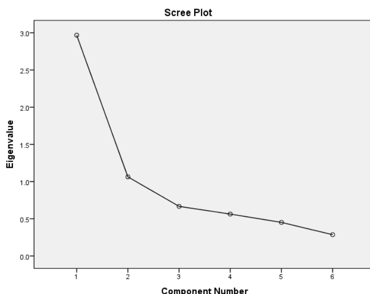
نمودار ۱- نمودار سنگریزه مقادیر ارزش ویژه هر یک از سوالات
